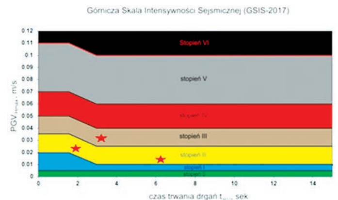
Rys. 4 Wykres intensywności drgań gruntu od wstrząsu z 13.01.2020 r. zarejestrowanego na stanowiskach AMAX w Orontowicach, w Chudowie w rejonie szybu VI oraz w Bujakowie
