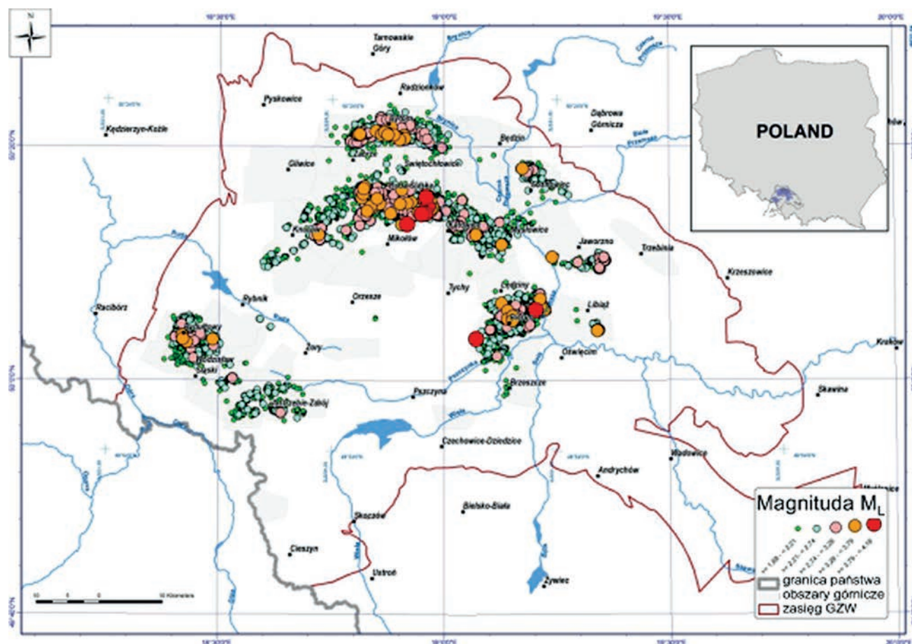
Rys. 1 Położenie ognisk wstrząsów w GZW w latach 1977–2019
