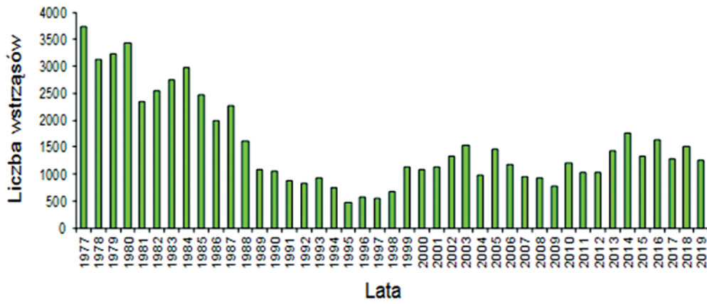
Rys. 2 Zestawienie liczby wstrząsów w GZW w okresie 1977–2019
